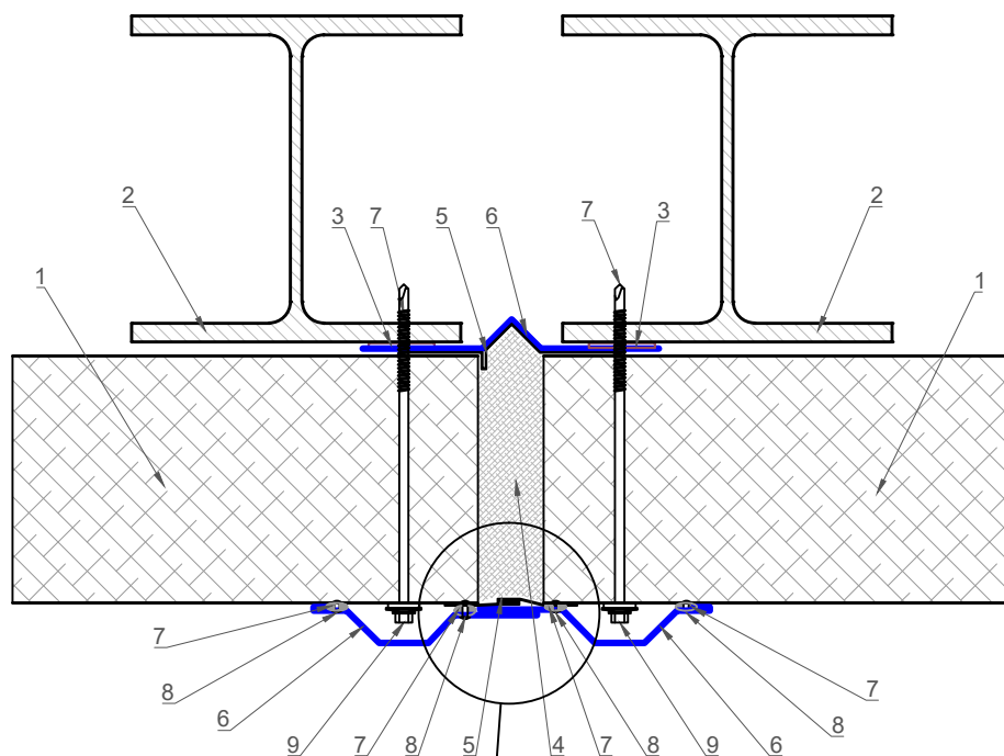
Узел А (3:1)
