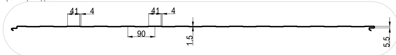
Трапецивидная ПХ
