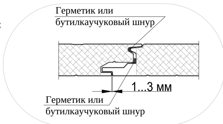
Рисунок 5. Виды профилирования внутренней обшивки сэндвич-панелей ПСТ Z и ПСТ SF, размеры указаны в мм
