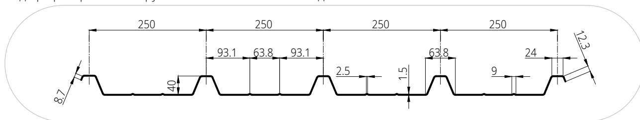
Рисунок 10. Вид профилирования наружной обшивки обшивки сэндвич-панелей ПКТ Z
