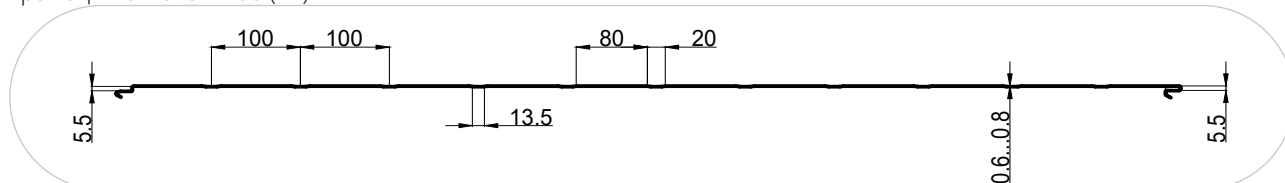
Трапеция с шагом 100 (Т1)
