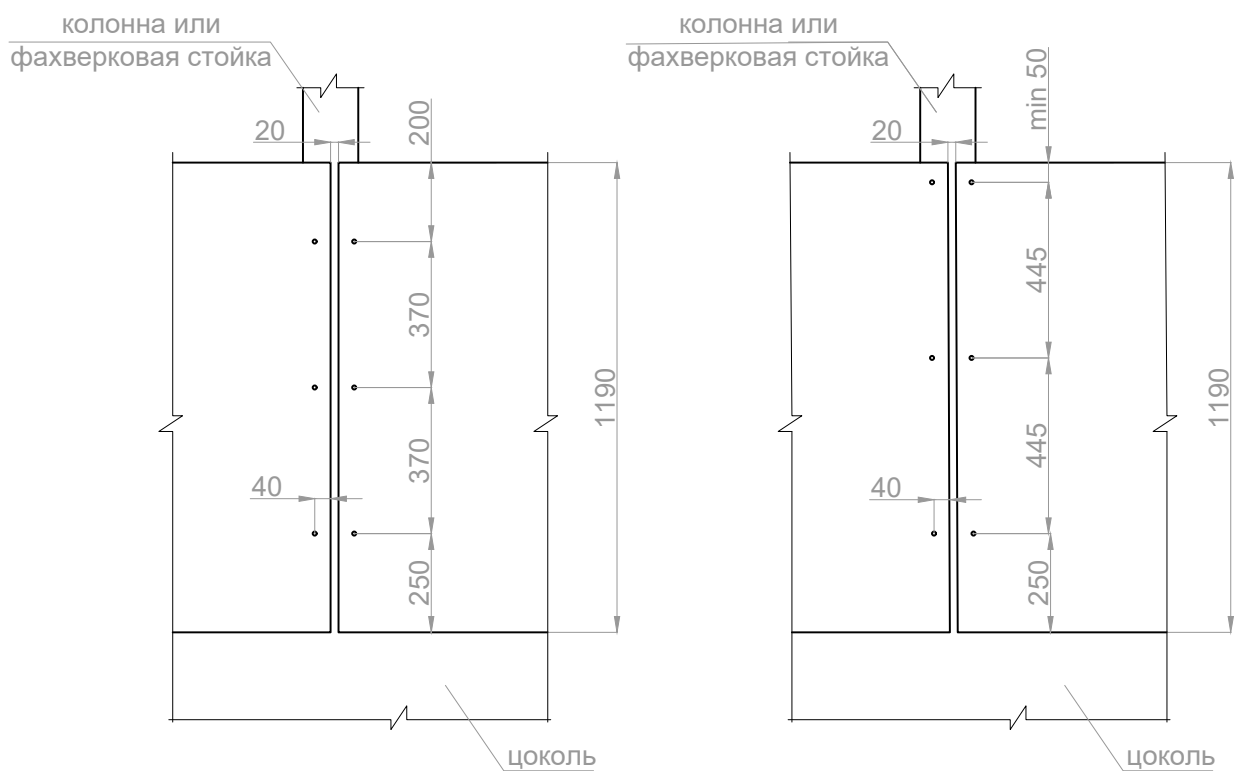
Рисунок 14. Стеновые панели ПСТ Z первого ряда. Варианты крепления к колонне или фахверку при горизонтальной раскладке
