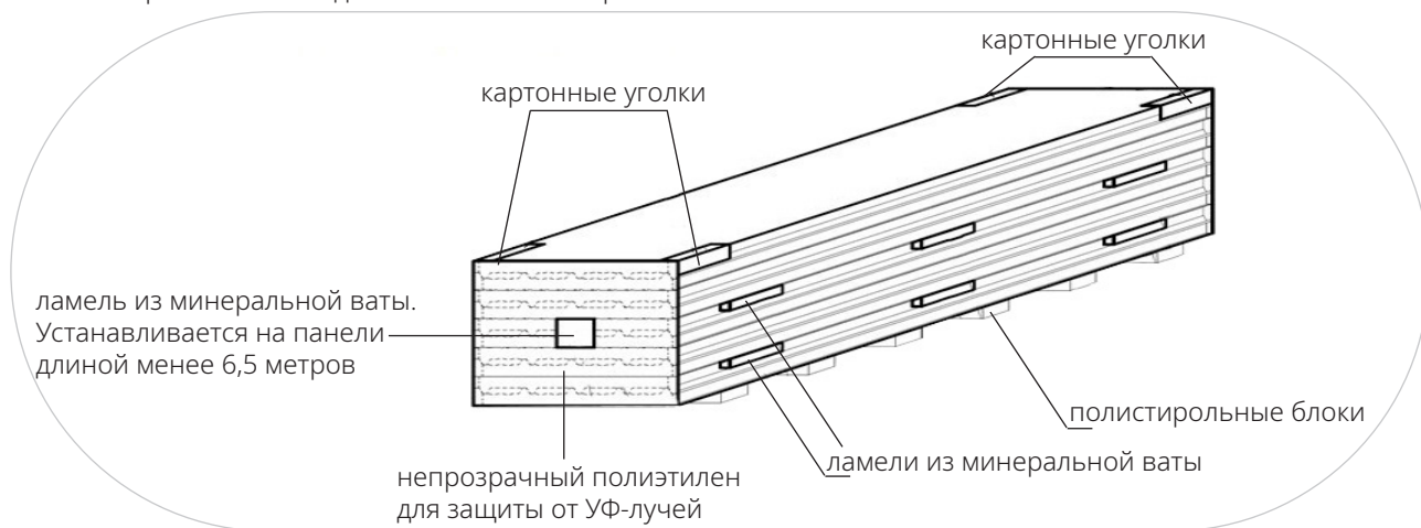
Рисунок 13. Упаковка кровельных сэндвич-панелей с минеральной ватой
