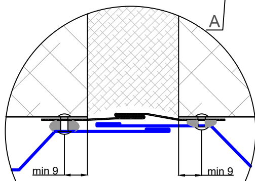
Узел А (3:1)
